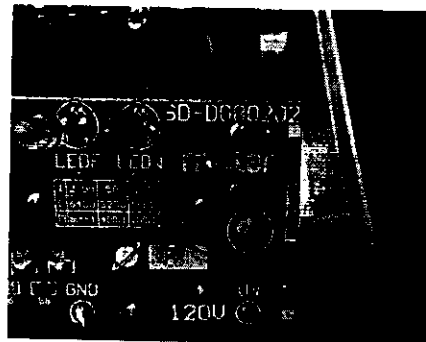
TARJETA(S) ELECTRÓNICA(S) DETERIORADO (Presenta una coloración oscura a la altura del circuito de tensión)
