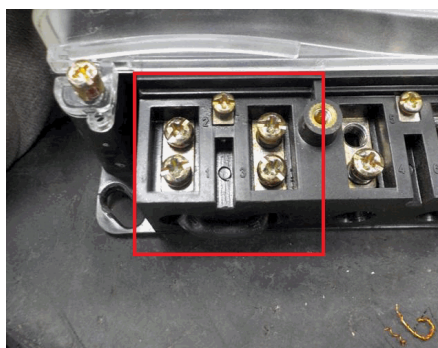
BLOQUE DE TERMINALES CON ELEMENTO EXTRAÑO (Conductor entre los terminales de entrada y salida de fase )
