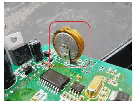
TARJETA(S) ELECTRÓNICA(S) DETERIORADO (Elemento de estado sólido C1)
