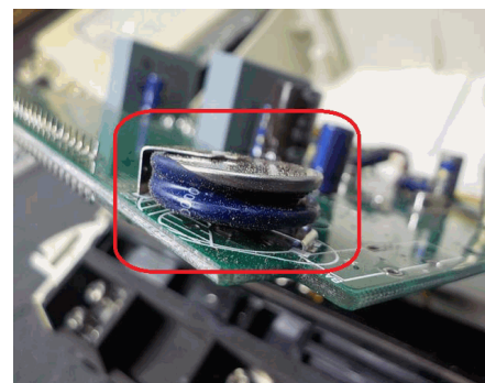
Tarjetas electronica ROTO (Elemento de estado solido C10)
