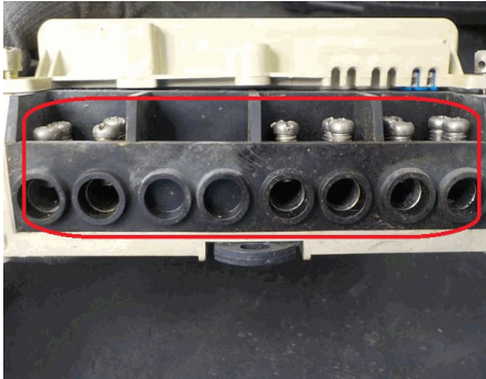
BLOQUE DE TERMINALES DETERIORADO (Terminales y tornillos sulfatados)
