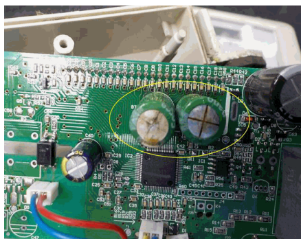
TARJETA(S) ELECTRÓNICA(S) DEFORMADO (Elementos de estado solido C64 y C46 deformados)
