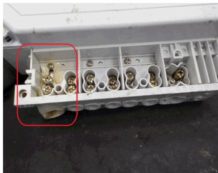
BLOQUE DE TERMINALES QUEMADO (Terminal entrada de fase R)
